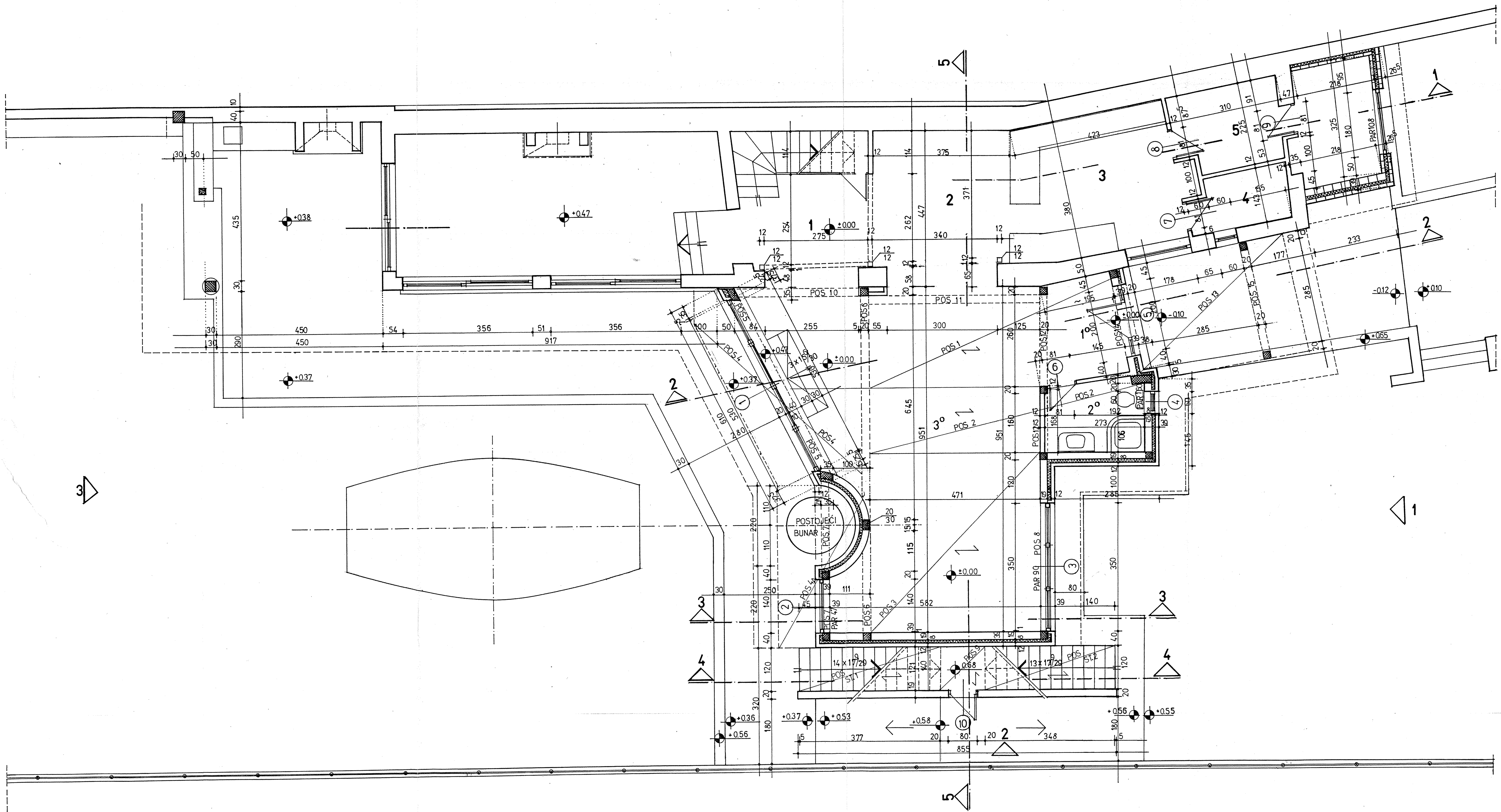
OSNOVA PRIZEMLJA
